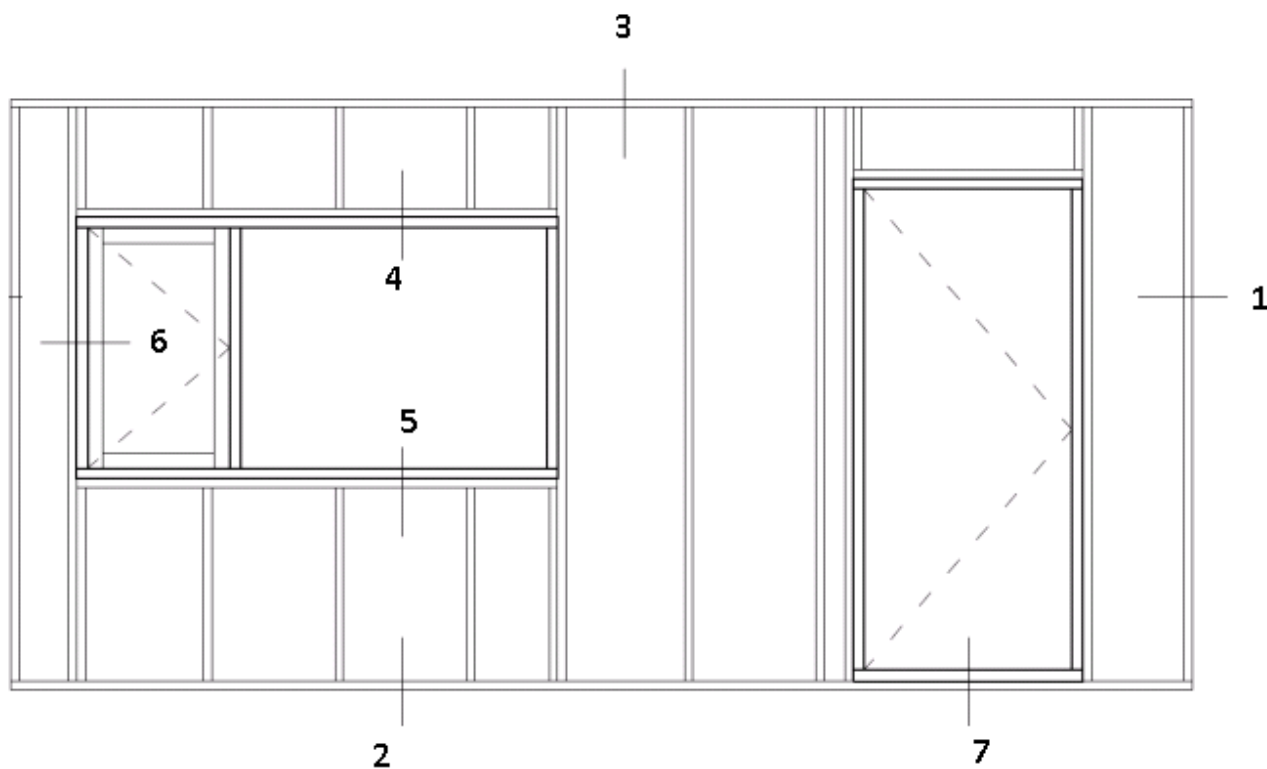
Bijlage 2 details binnenspouwbladen
